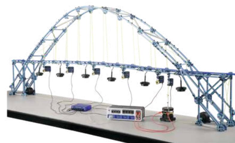
Experimento de vibración de puente Cod. EX-5548
