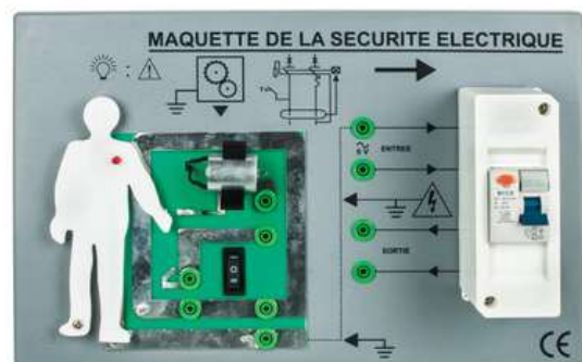
Demostración del disyuntor Cod. CBD17
