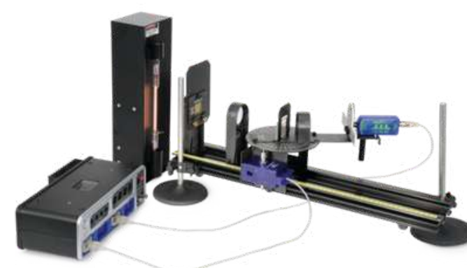
Experimento de espectro atómico Cod. EX-5546B
