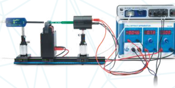
Experimento de efecto Hall Cod. EX-5560
